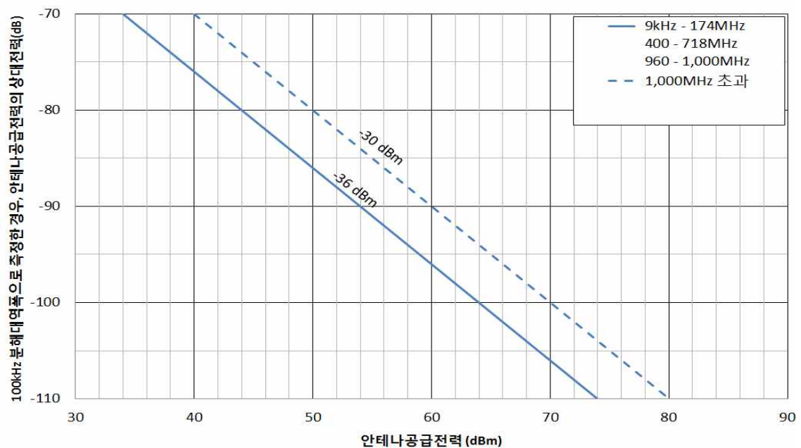
스퓨리어스영역 불요발사의 허용범위(분해대역폭 100 kHz)
